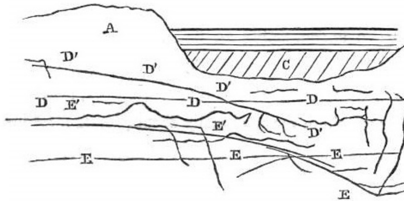
Fig. 2. Ajuste isostático propuesto por Herschel (1836).
