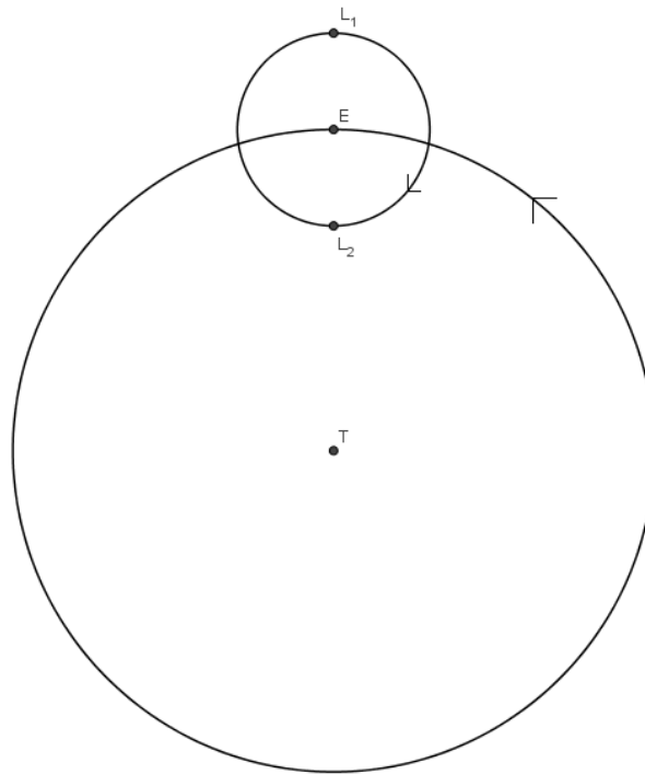
2. Diagrama del movimiento entre el primer par de eclipses.
