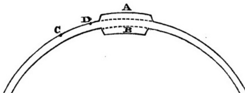
Fig. 1. Modelo de compensación isostática de Airy (1855).
